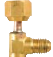
1/4"フレアオス
