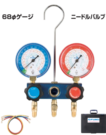
68φゲージ付ニードルバルブマニホールドキット
