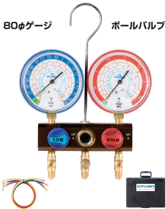
80φゲージ付ボールバルブマニホールドキット
