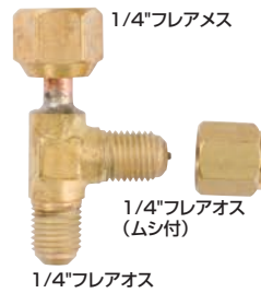
1/4"フレアオス
