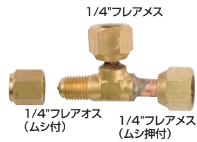
1/4"フレアメス
